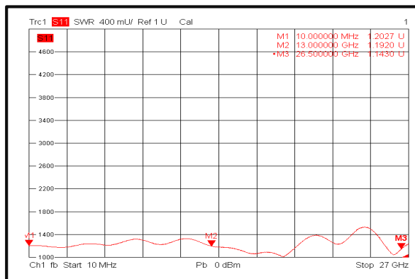
VSWR @-40°C
